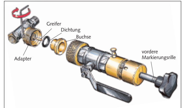
Demontageblock (Best.-Nr. 013G3086)
